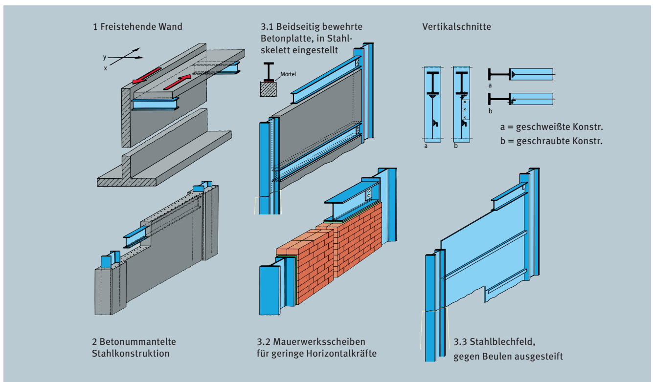
Bild 1: Schubsteife Wandscheiben - Ausführungsvarianten
