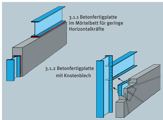
Bild 2: Schubübertragung Platte - Stahltragwerk
